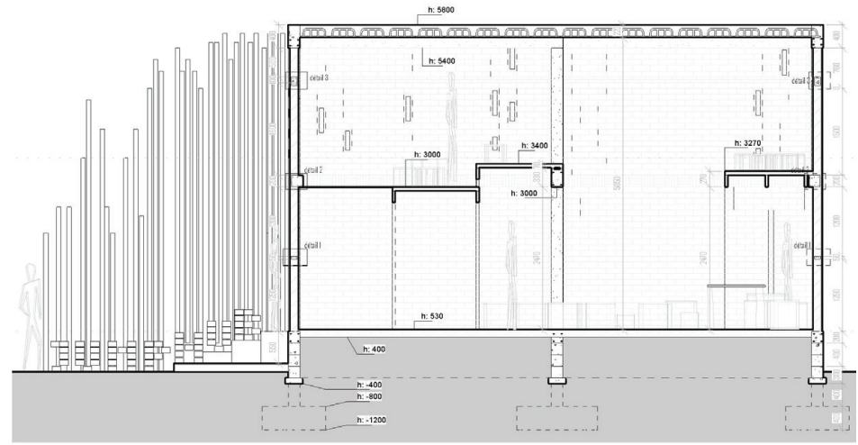
COUPE A-A
