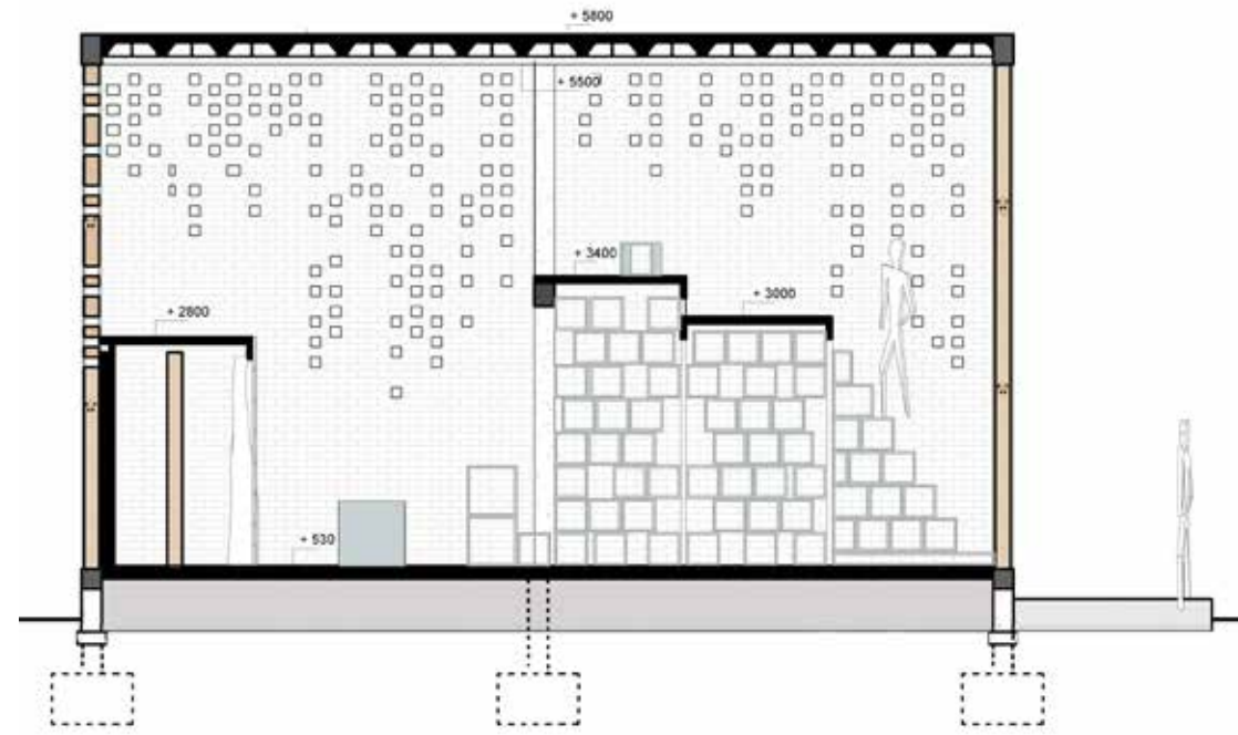
COUPE B-B
