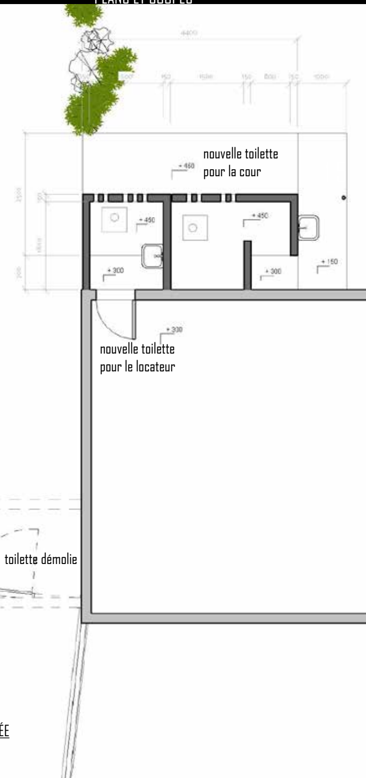
PLANS ET COUPES
