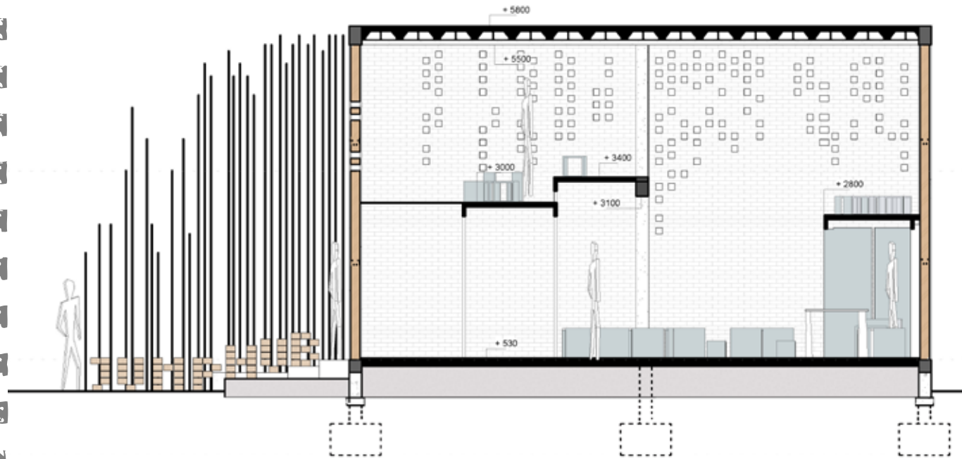
COUPE A-A
